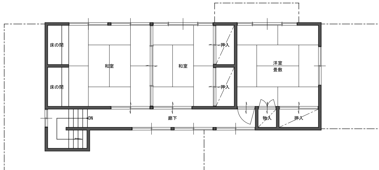
2 階 平 面 図
